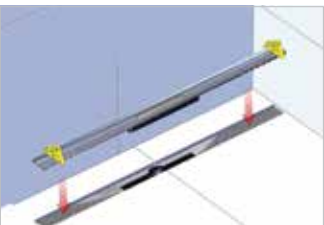
Kapak altına Yapıştırıcı sürerek klavuz yardımı ile kapağı yerleştiriniz. Patentli ters açılı kanallar kilitlenmeyi sağlayacaktır. Apply adhesives under cover, place the cover on. ( with guide ) Patent reverse angled channels it will provide deadlock.
