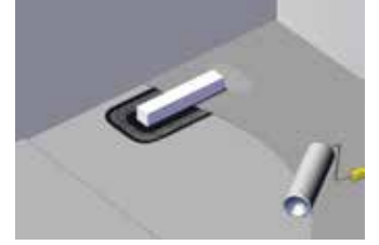
Duş alanına min. 2 kat sürme izolasyon ile yalıtım yapınız. Insulate the shower area min. 2 layer With sliding isolation.
