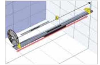
Kapağı klavuz yardımı ile alan uzunluğuna göre kesiniz. Cut Cover by length of the field. ( with guide )
