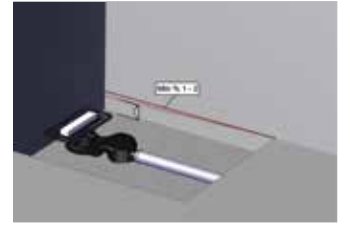
Alt sifon grubunu tesisata bağlayınız. ( Yan Çıkış EN 50 ) Connect the plumbing ( Side Outlet / EN 50 )
