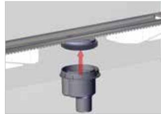
Alt çıkış sifon bağlantısında fermatür ve kova aynı hizaya gelmelidir. Oder Part and siphon must come into same line.
