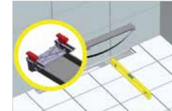
Koruyucu stroforu çıkarak metal çerçeveyi kademeli ayar parçalarının kodunu terazi ile her noktadan ayarlayınız. Remove the protective styropor and adjust the level gradual parts from each point.
