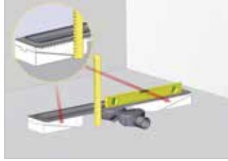
Yükseklik ayar setini zemin kotuna göre terazi ile ayarlayınız. Her kademe 2 mmdir. Adjust height adjusting set with scale according to the ground level. Each step is 2mm.
