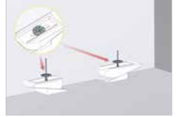
Özel strafor dubeliyle ayar setini sabitleyiniz. Fix the adjusting set with special styropor dowel. (opsiyonel)
