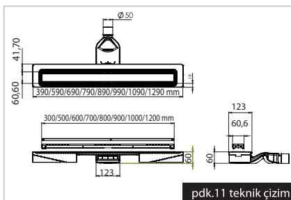
pdk.11 teknik çizim
