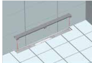
Koruyucu stroforu çıkarak metal çerçeveyi yerleştiriniz. Remove the protective styropor and place the metal sash.
