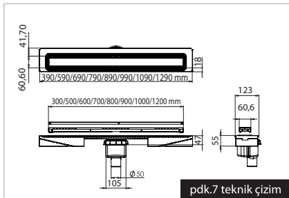
pdk.7 teknik çizim
