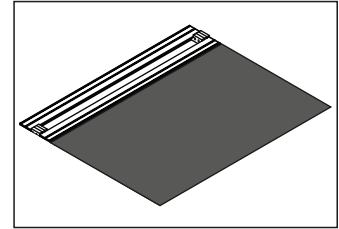
Düzeltilme betonunun meyilini duş kanalına doğru min %1 eğimle veriniz.
