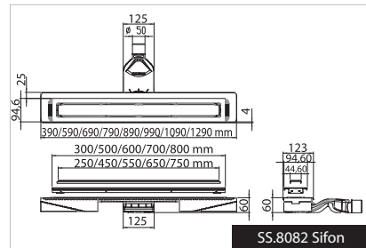
SS.8082 Sifon
