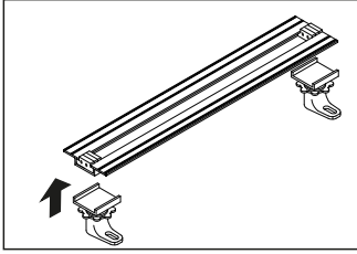
Yükseklik ayar parçasını gövdeye yerleştirin.
