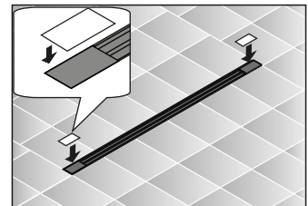
Sabitleme kapaklarını ayarlama işleminden sonra tekrar takın ve ardından kapağı yerleştirin.
