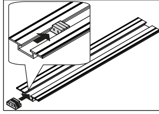
Sızdırmazlık parçalarını kanal alanına yerleştirin.
