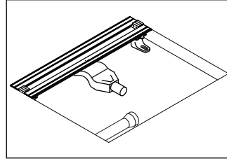
Linear Kanalı zemine yerleştirin.
