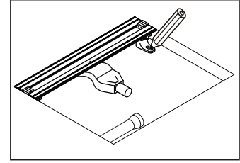
Yükseklik ayar setini ayarlayın. Noktaları zemin seviyesine göre işaretleyin.
