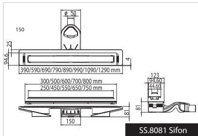
SS.8081 Sifon
