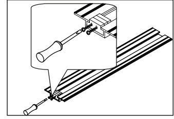
Sızdırmazlık parçalarını vidalayın.
