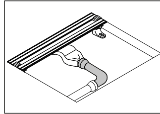
Duş kanalını tesisata bağlayın ve koruyucu straforu tıkanmaya karşı yerleştirin.
