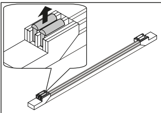
Koruyucu straforu kaldırın ve kademeli parçaların seviyesini her noktadan ölçek ile ayarlayın.
