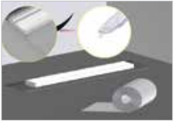
Düzeltme betonuna astar sürünüz. İzolasyon bandını metal-beton birleşimine yapıştırınız.
