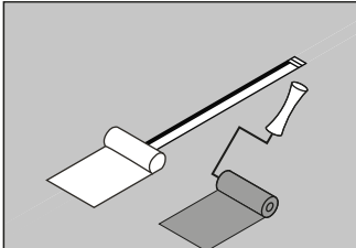
Düzeltilme betonuna astar sürünüz. İzolasyon bandını metal-beton birleşimine yapıştırınız.
